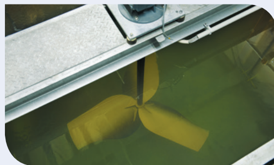
Rührwerk im Reifebecken
