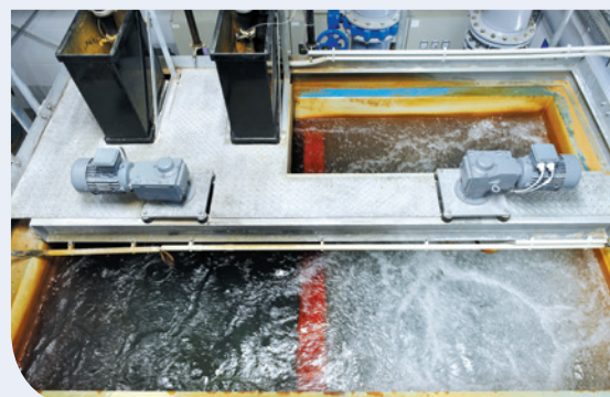
Rührwerk im Koagulationsbecken
